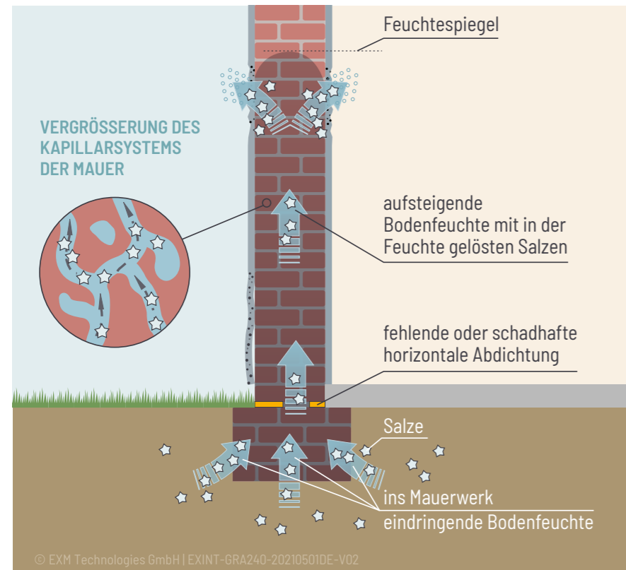
GRAFIK 01: Aufsteigende Bodenfeuchte, mittransportierte bausubstanzschädigende Bodensalze
